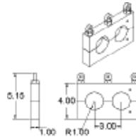
AVSC Clamps
